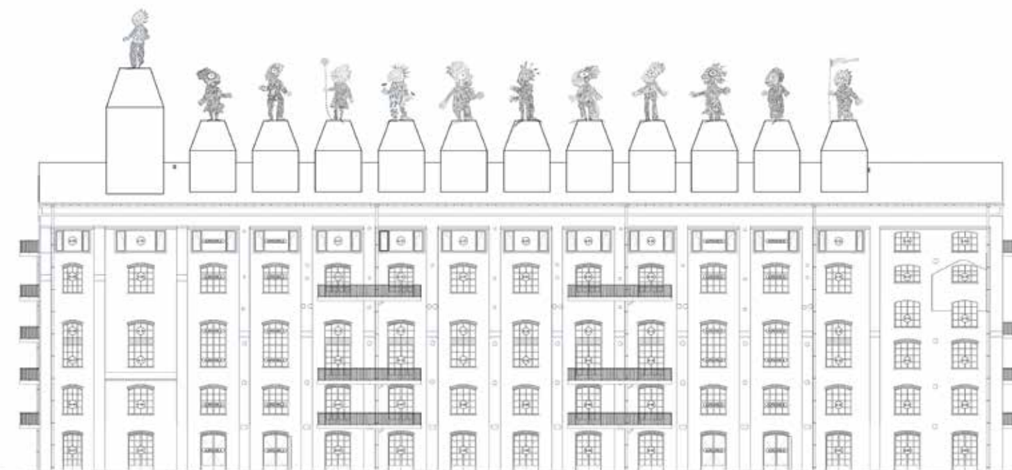
ANSICHT NORDEN
